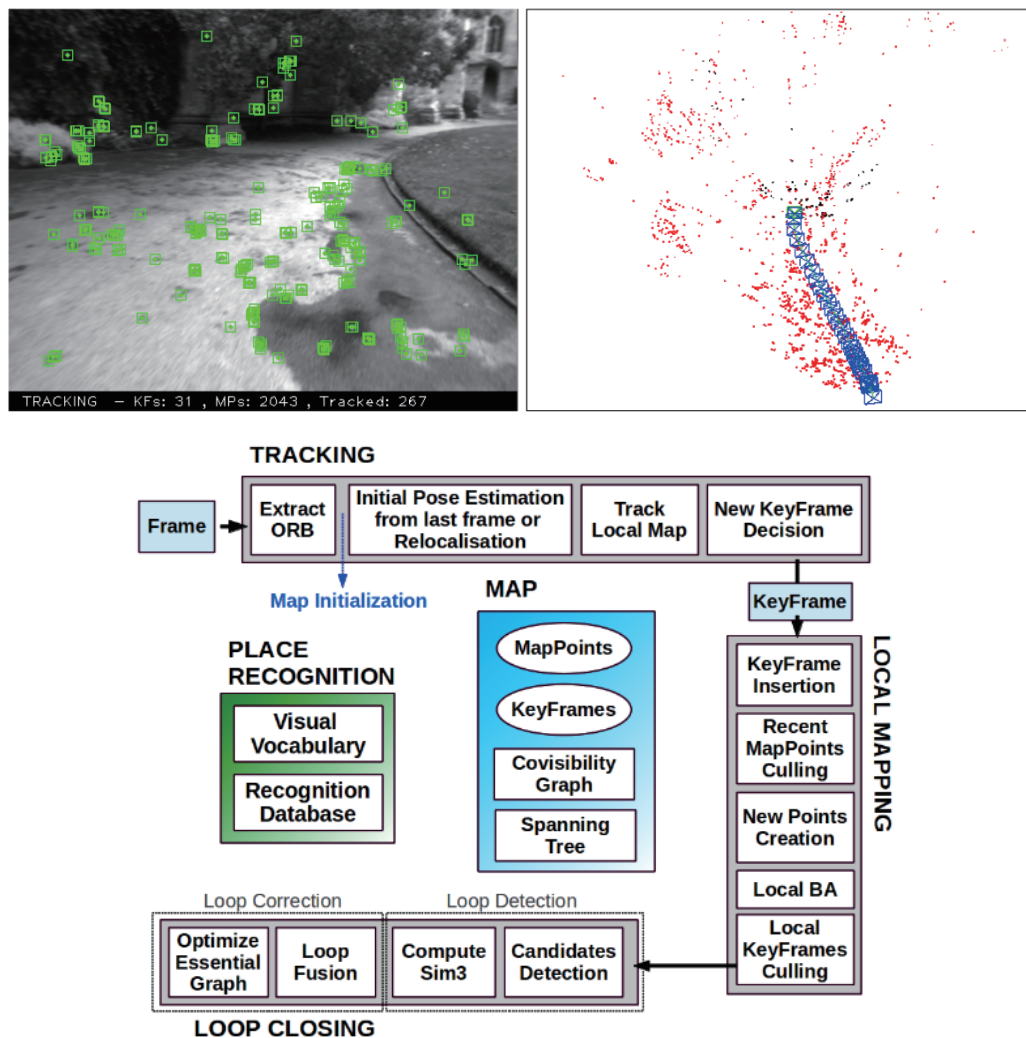
图 14-3 ORB-SLAM 运行截图。左侧为图像与追踪到的特征点，右侧为相机轨迹与建模的特征点地图。下方为它标志性的三线程结构。
