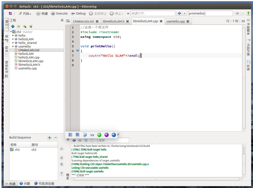
图 2-12 Kdevelop 界面。
